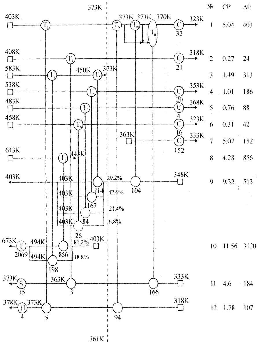
Рис. 3 – Сеточная диаграмма проекта реконструкции теплообменной сети СПЦ с разделением на пинче, построенная для \Delta T_{\min} = 12\text{K} . T_1 - T_{11} – рекуперативные теплообменные аппараты; C – утилитные теплообменные аппараты; F – трубчатая печь; S – нагрев парами среднего давления; CP – потоковая теплоемкость, кВт; № – номер потока из таблицы 1. Под обозначение теплообменных аппаратов показаны их тепловые нагрузки, кВт; на расщеплениях потоков показаны проценты от общего массового расхода потока. На штриховой линии, разделяющей полную систему на тепловой сток и тепловой источник показаны пинч-температуры
