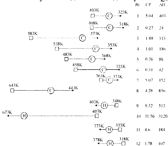
Рис. 1 – Сеточная диаграмма существующей тепло-обменной системы процессов дистилляции каменноугольной смолы и переработки нафталиновой фракции. Поток, направленный направо – горячие потоки, налево – холодные; С – охлаждение, Н – нагрев
