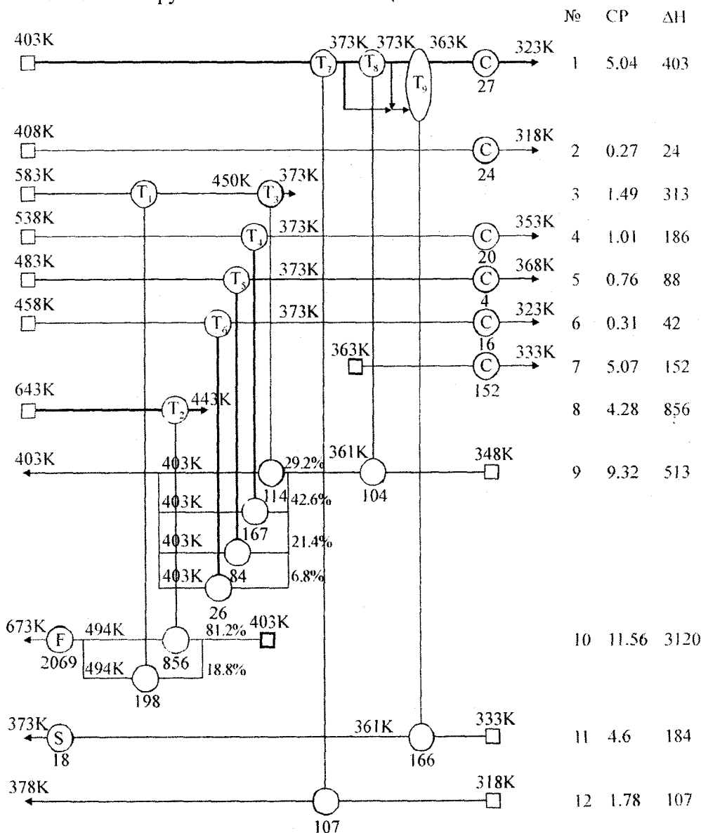
Рис. 4 – Сеточная диаграмма оптимизированного проекта реконструкции теплообменной сети СПЦ. Обозначения аналогичны обозначениям на рис. 3
