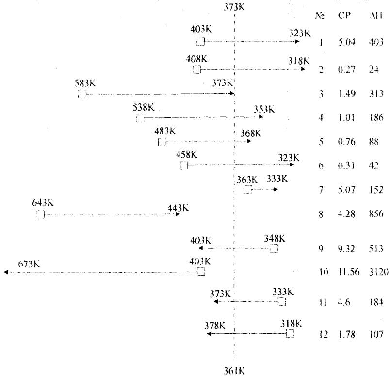
Рис. 2 – Полная система технологических потоков СПЦ, участвующих в интеграции. Пунктирная линия – разделение на пинче. Горячие потоки направлены направо, холодные – налево. № – номер потока по таблице 1; CP – потоковая теплоемкость, кВт/К; \Delta H – изменение потоковой энтальпии, кВт
